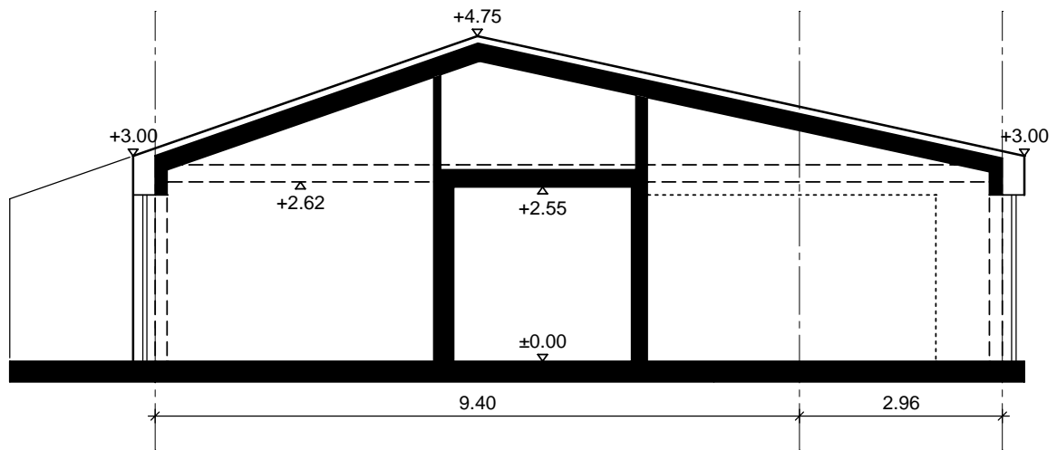
Prinzipialschnitt
